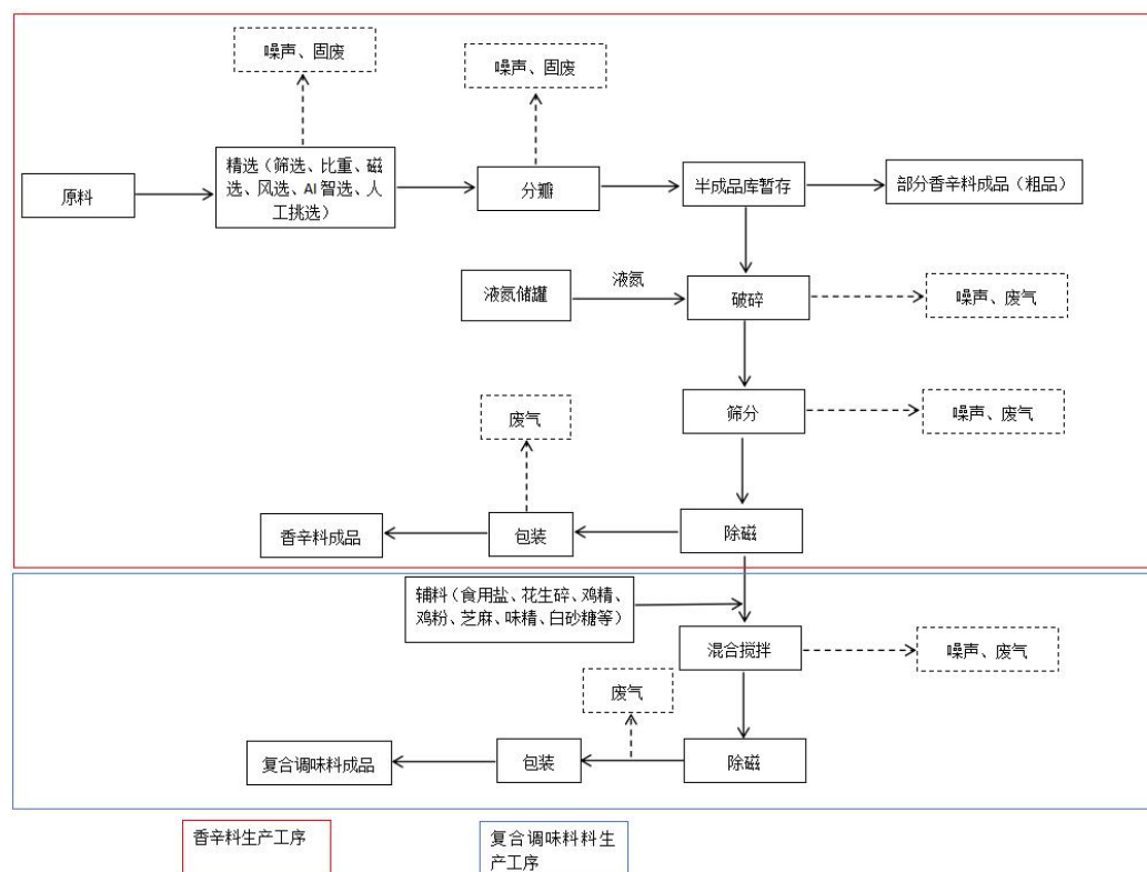
图 5 雪麦龙调味料生产线建设项目生产工艺及污染物产生流程图
