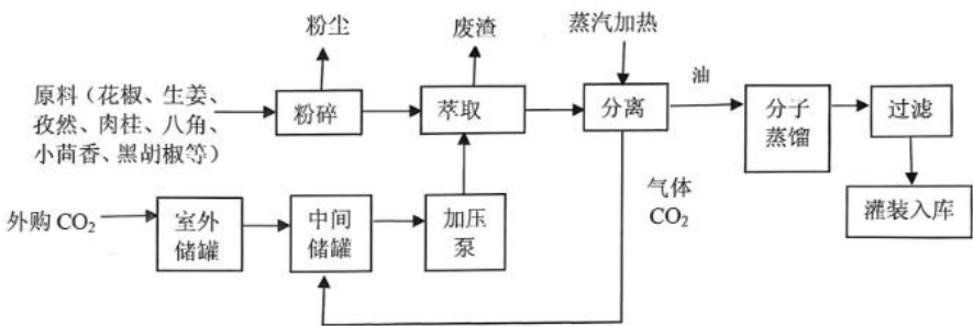
(1) 天然植物精油生产工艺流程图：
