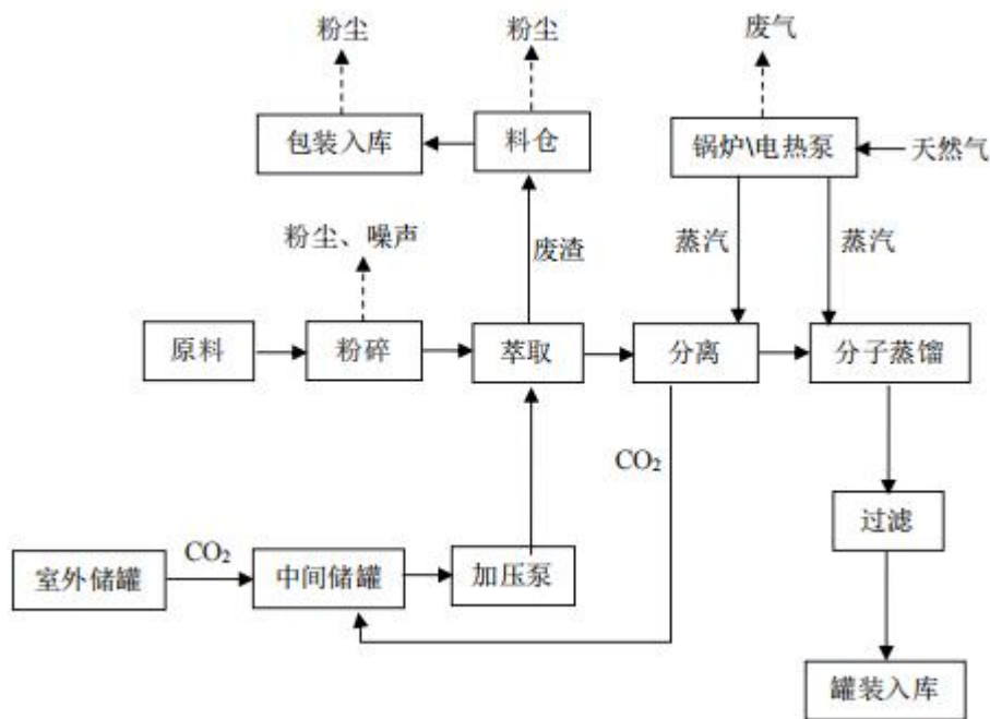
图 4 天然植物香料油建设项目生产工艺及污染物产生流程图
