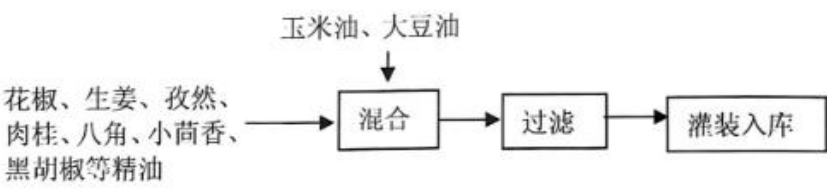
图2 年产15000吨天然植物香料油建设项目生产工艺及污染物产生流程图
