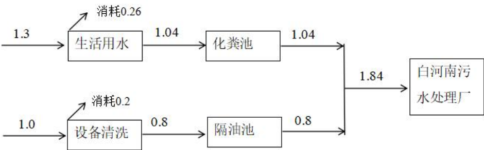
图 8 本次工程水平衡图 (m 3 /d)
