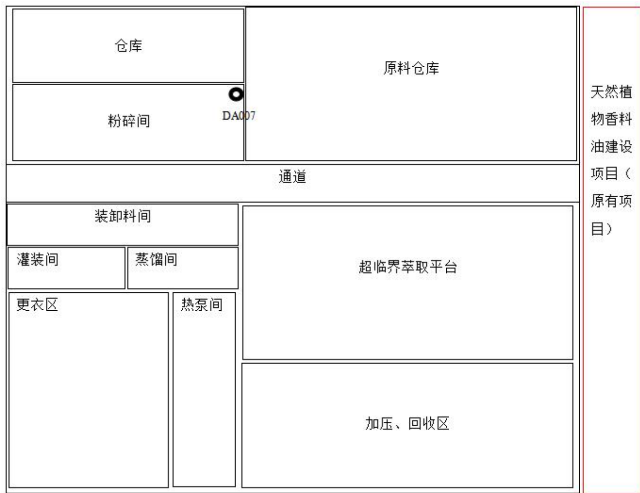
附图四 本次项目平面布置图
