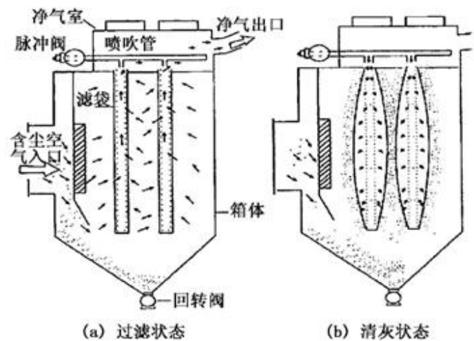
图 7 除尘器工作原理图
