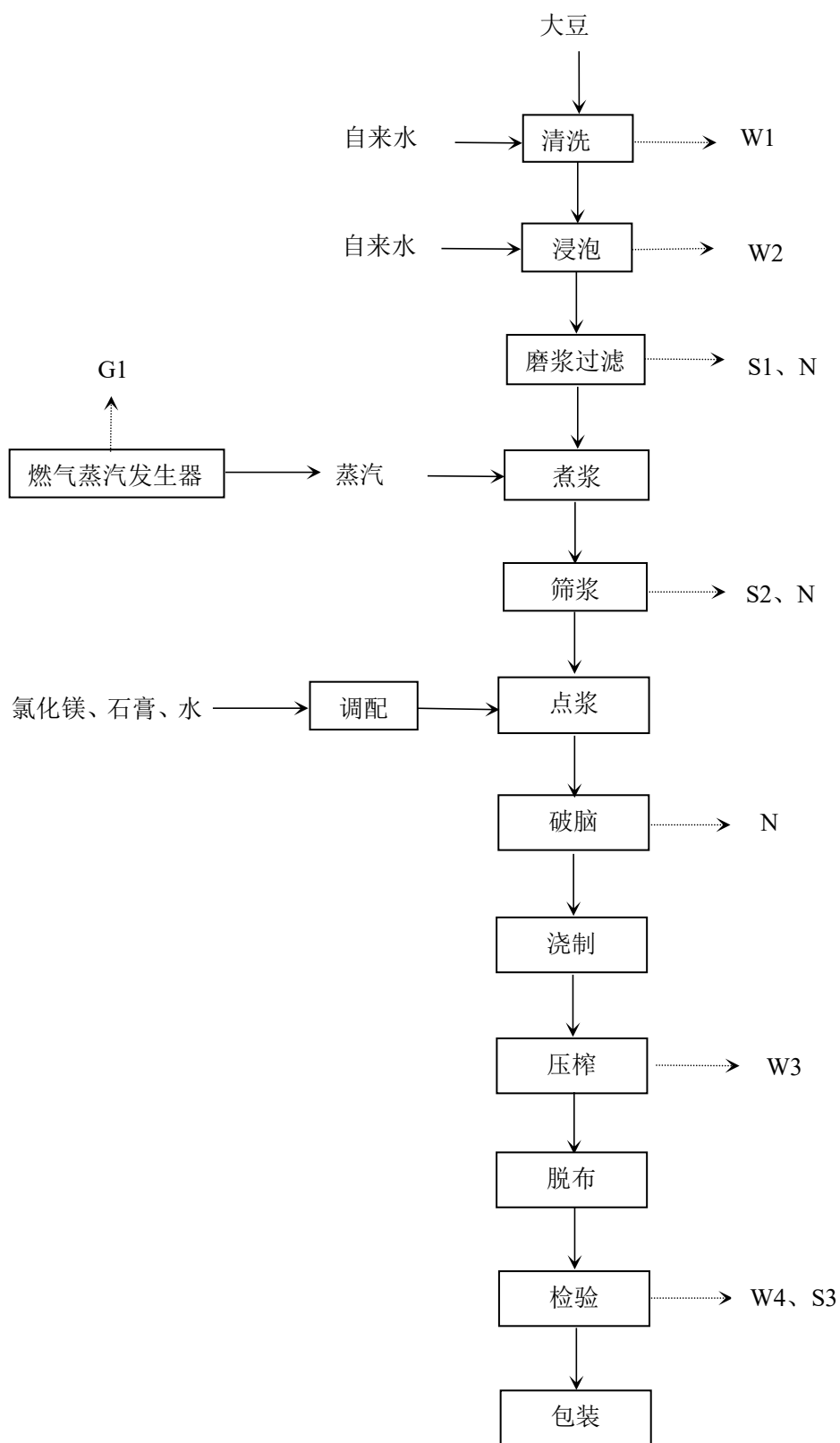
图3 本项目生产工艺流程及产污环节
