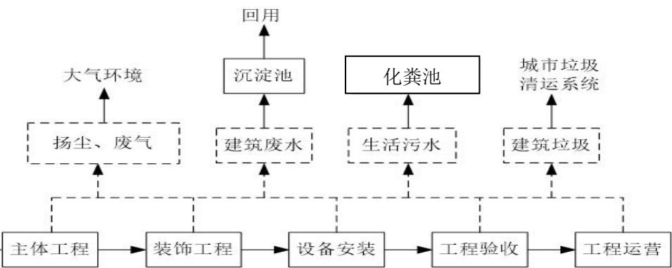
图 2 施工工艺流程及产污环节示意图
