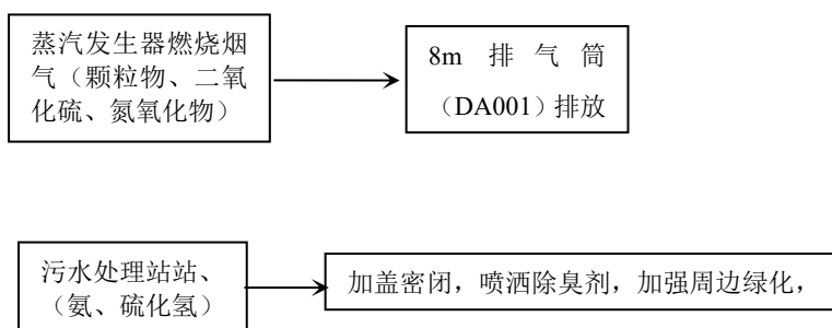
图 4 废气收集处理系统示意图
