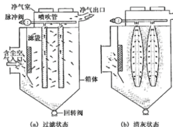
图3 除尘器工作原理图
