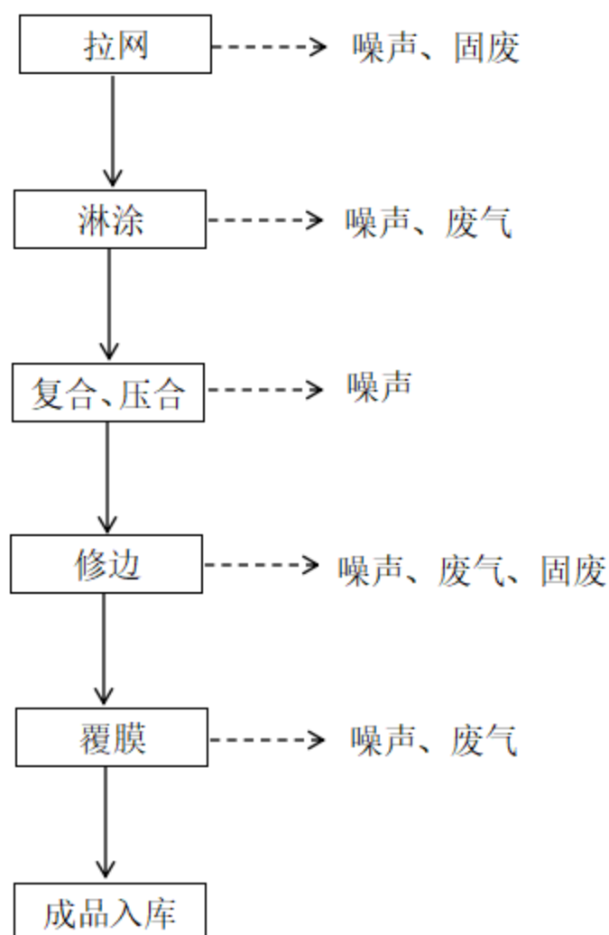
图 1 项目生产工艺及产污环节示意图
